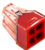
型号/Model: YL-604A 产品尺寸LxWxH: 19.5x13x13.1mm
