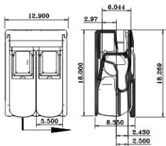
型号/Model: YL-PTC-212 产品尺寸LxWxH: 18.2x12.9x8.3mm
