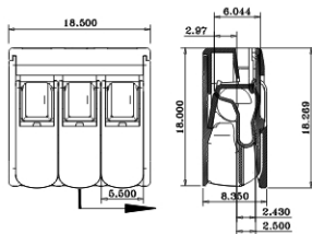
型号/Model: YL-PTC-213 产品尺寸LxWxH: 18.2x18.5x8.3mm
