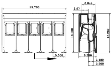
型号/Model: YL-PTC-215 产品尺寸LxWxH: 18.2x29.7x8.3mm
