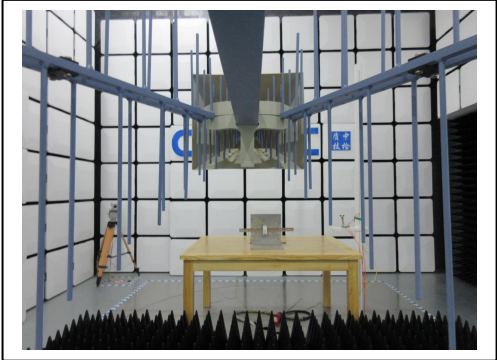
射频电磁场辐射试验
